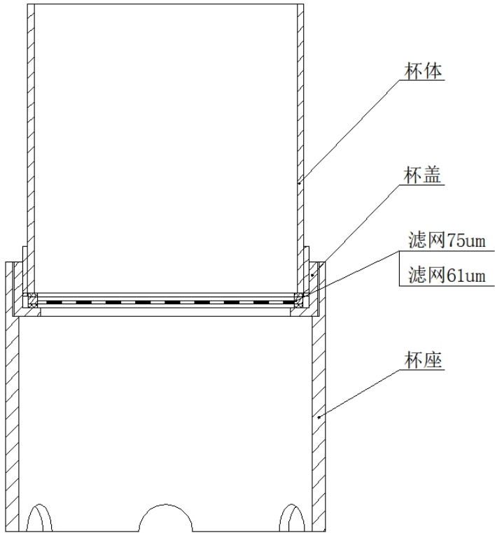
（图二）钻井液杯安装示意图
